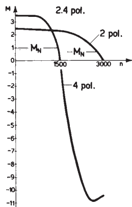
Motori autofrenanti a doppia polarità. Esempi di curve caratteristiche con andamento del momento di frenatura ipersincrona alla polarità alta.
