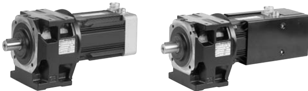
Esempi di servomotoriduttori coassiali con servomotore sincrono «brushless» e asincrono «vettoriale» cat. SR 04.
